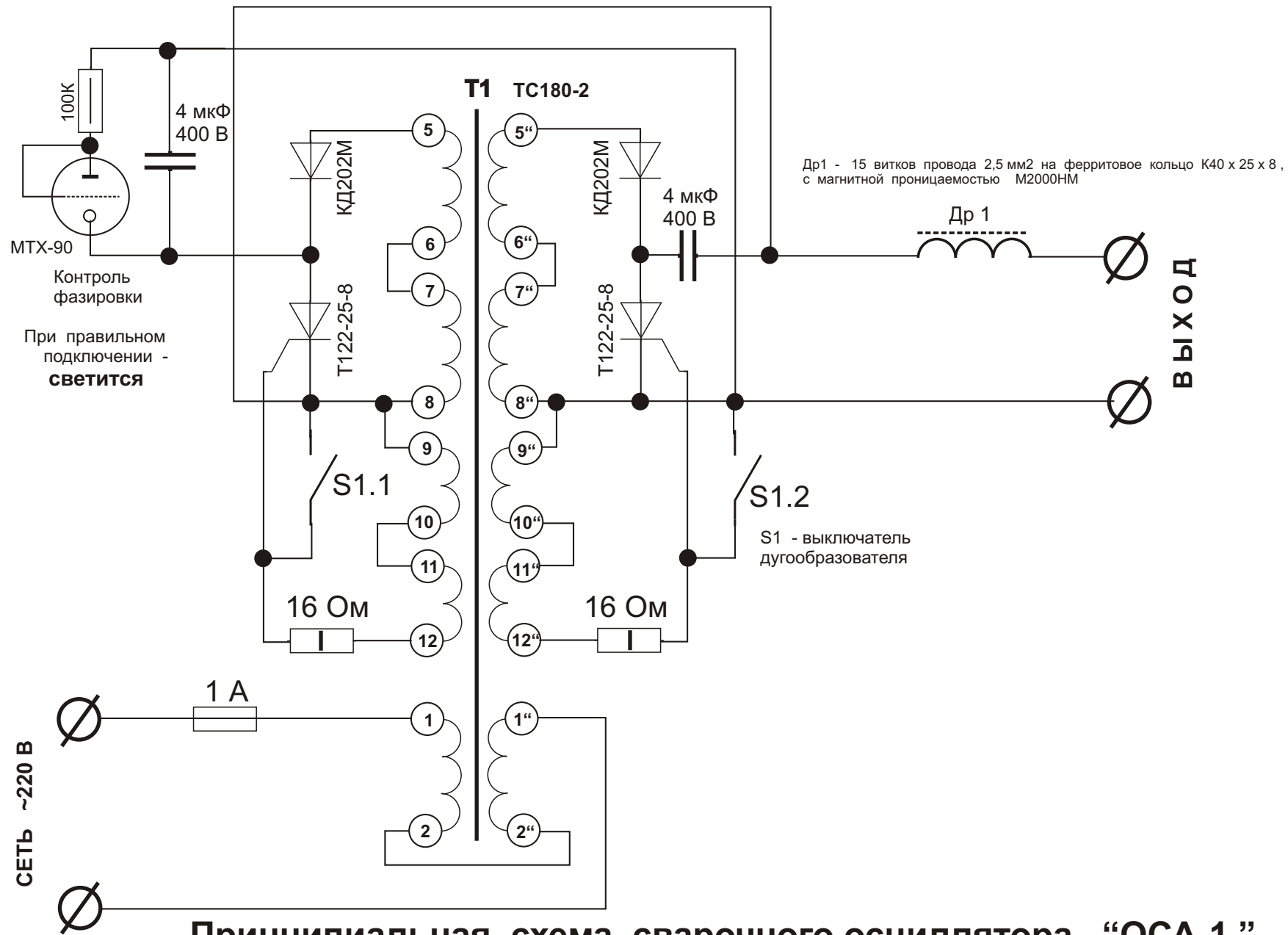
Принципиальная схема сварочного осциллятора "ОСА-1"
