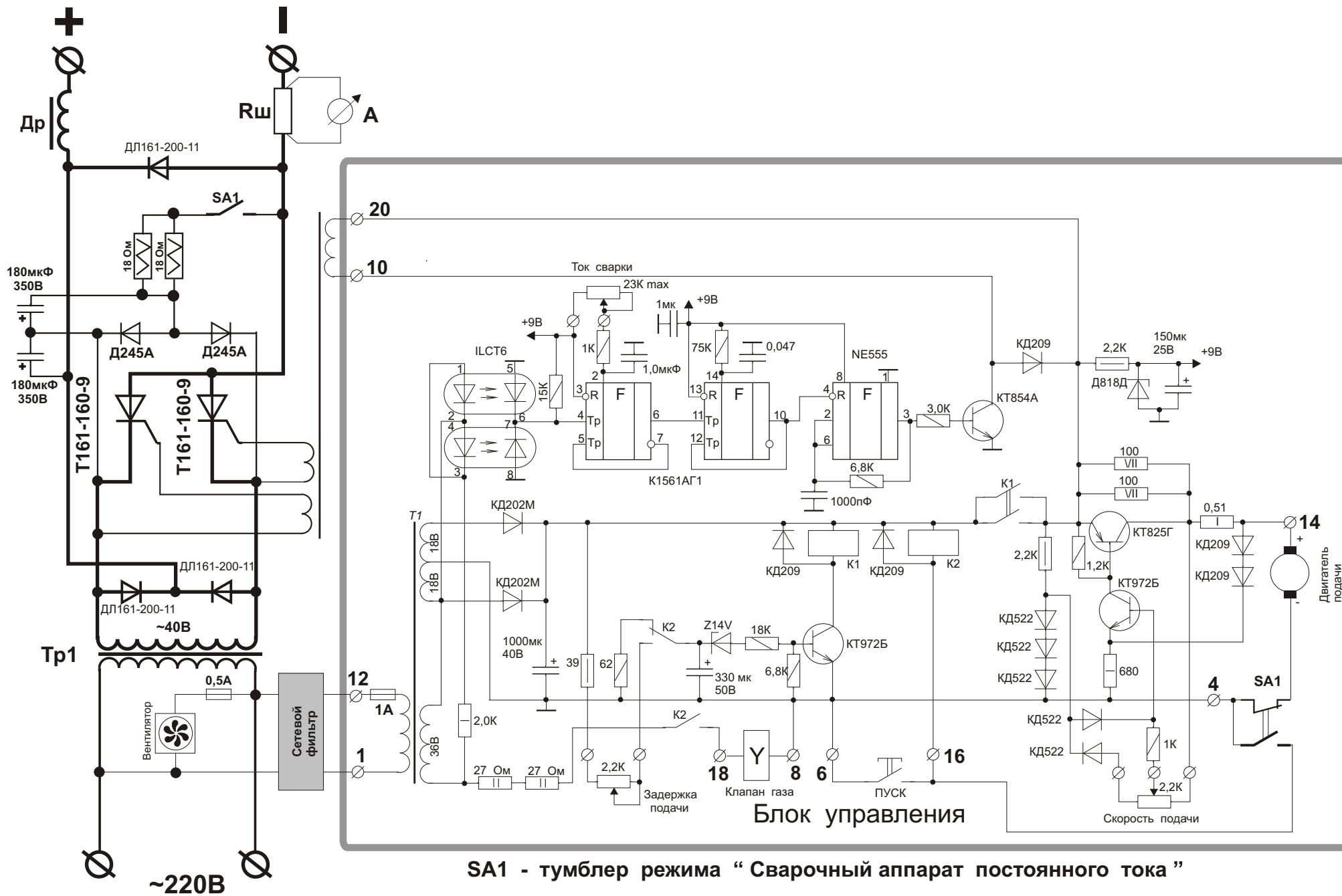
ПРИНЦИПИАЛЬНАЯ СХЕМА СВАРОЧНОГО ПОЛУАВТОМАТА
