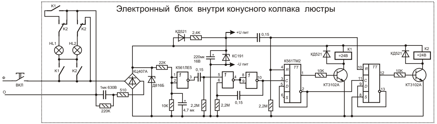
Принципиальная схема устройства управления лампами люстры
