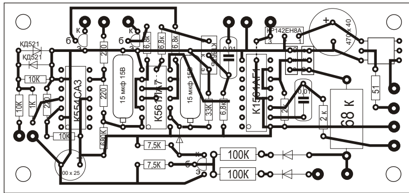
Печатная плата осциллятора ОСА-2
