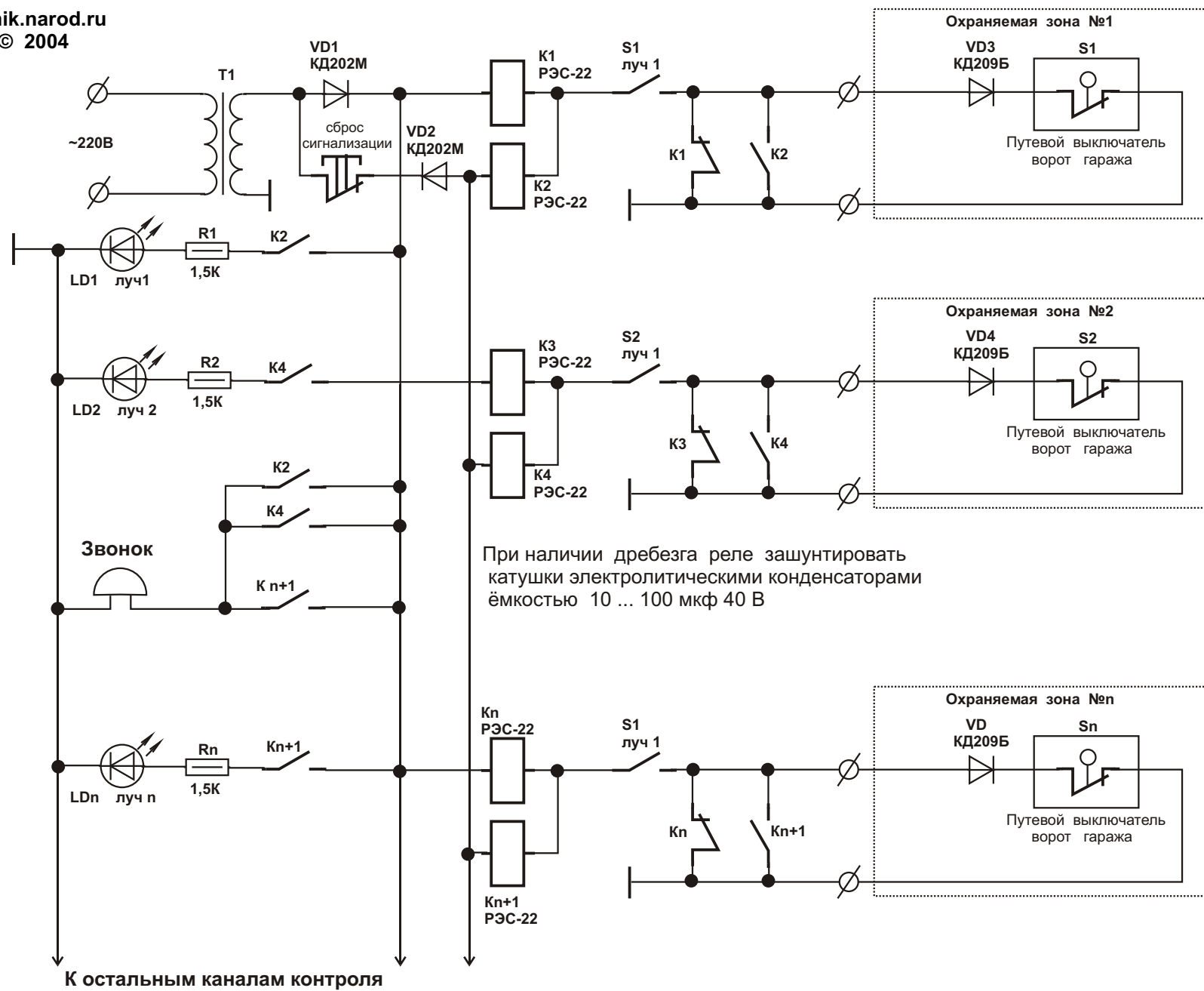
Принципиальная схема многоканальной охранной сигнализации
