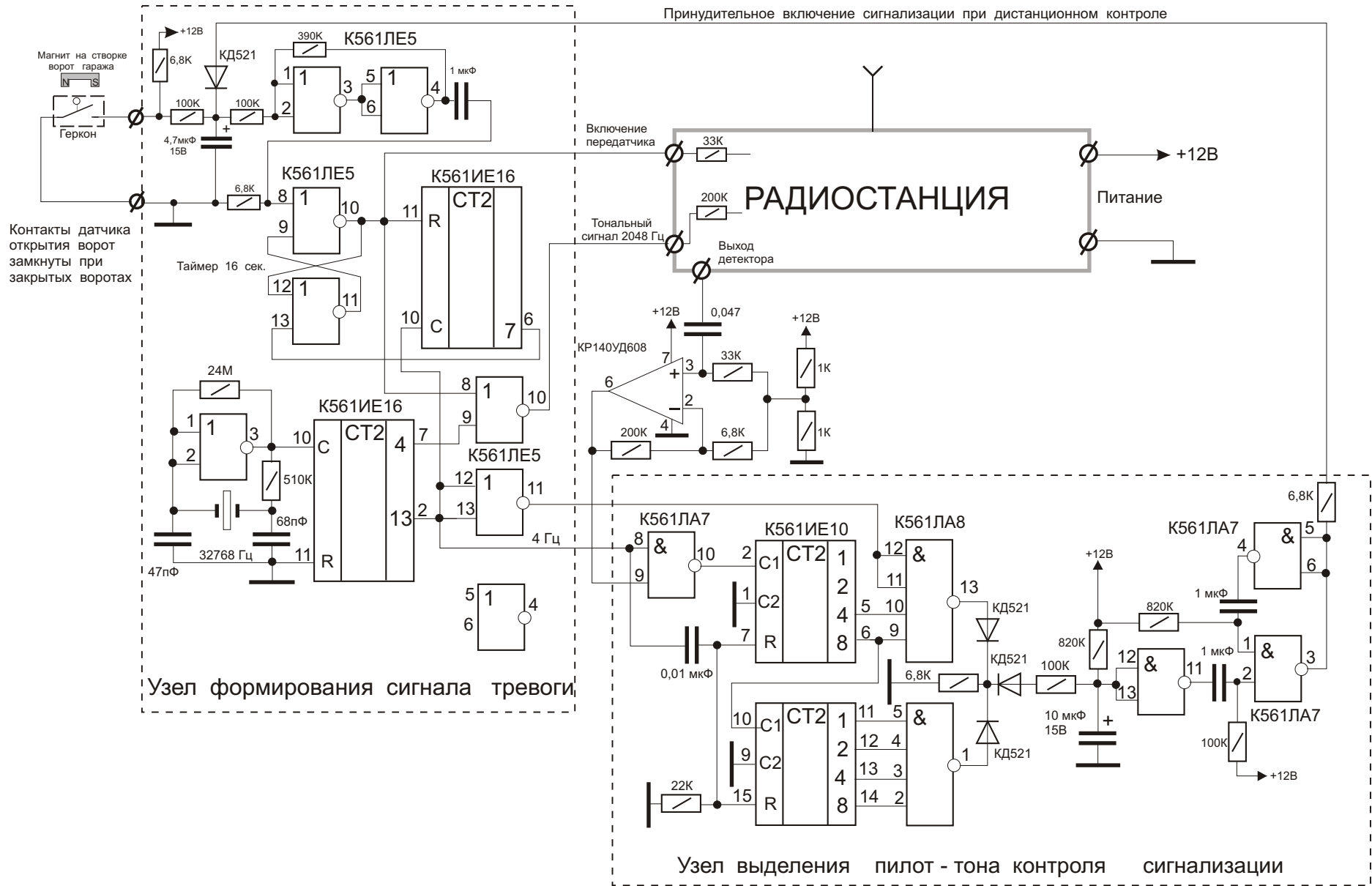
Принципиальная схема охранной сигнализации. Гаражный комплект.
